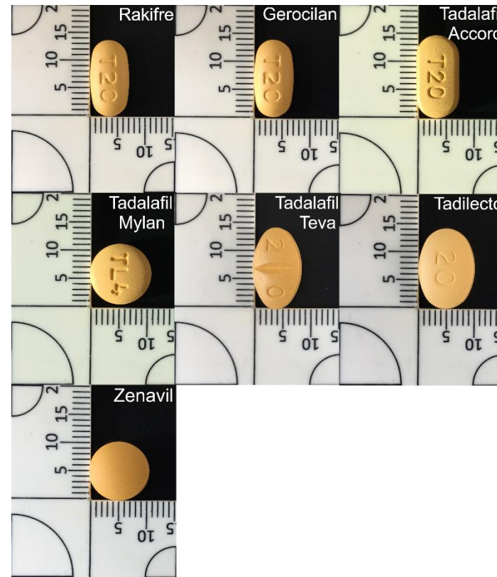
generic Cialis
