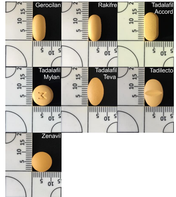
generic Cialis
